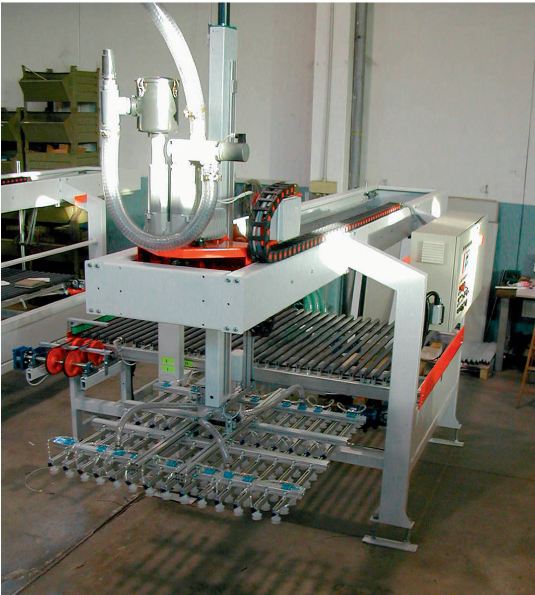
73) MCV – Macchina di carico/scarico a ventosa.
