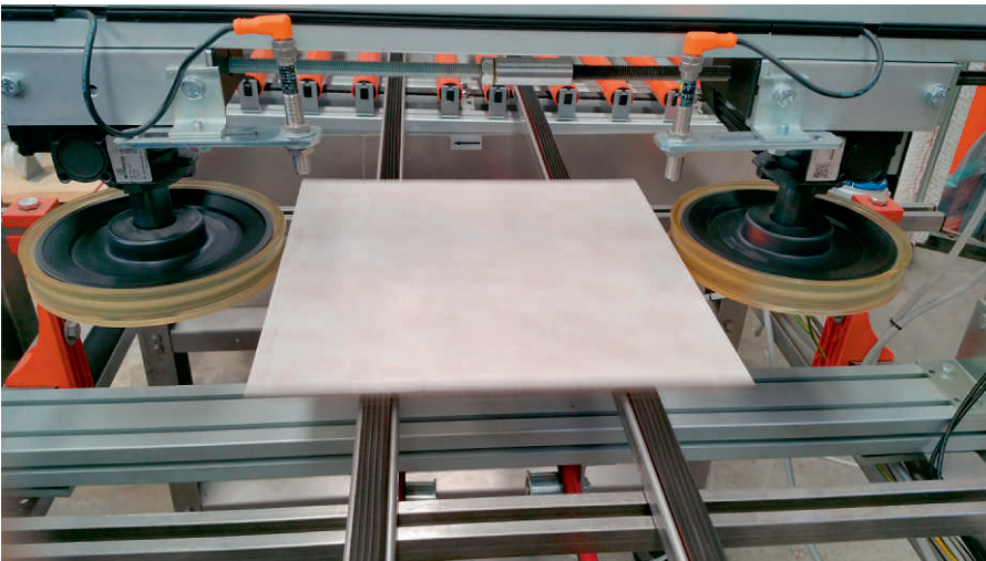
78) PP – Pareggiatore di piastrelle con fermo meccanico a ruota. 78) PP - Tile centring unit with mechanical wheel backstop.
